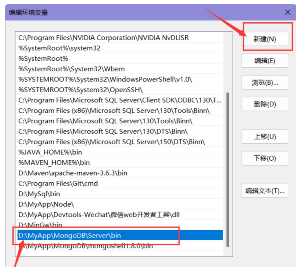
图 2.21 环境配置
