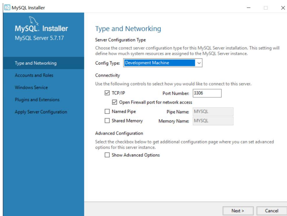
图 2.6 MySQL 配置
