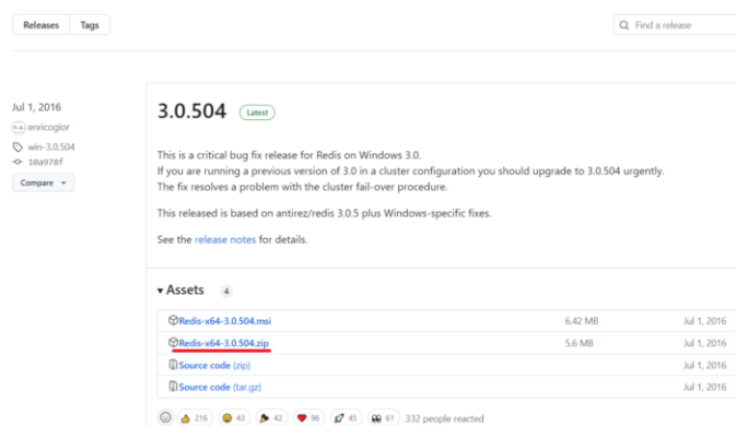
图 2.25 Redis 下载
