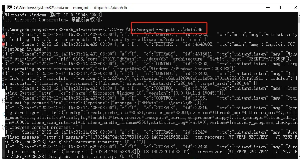
图 2.23 MongoDB 启动
