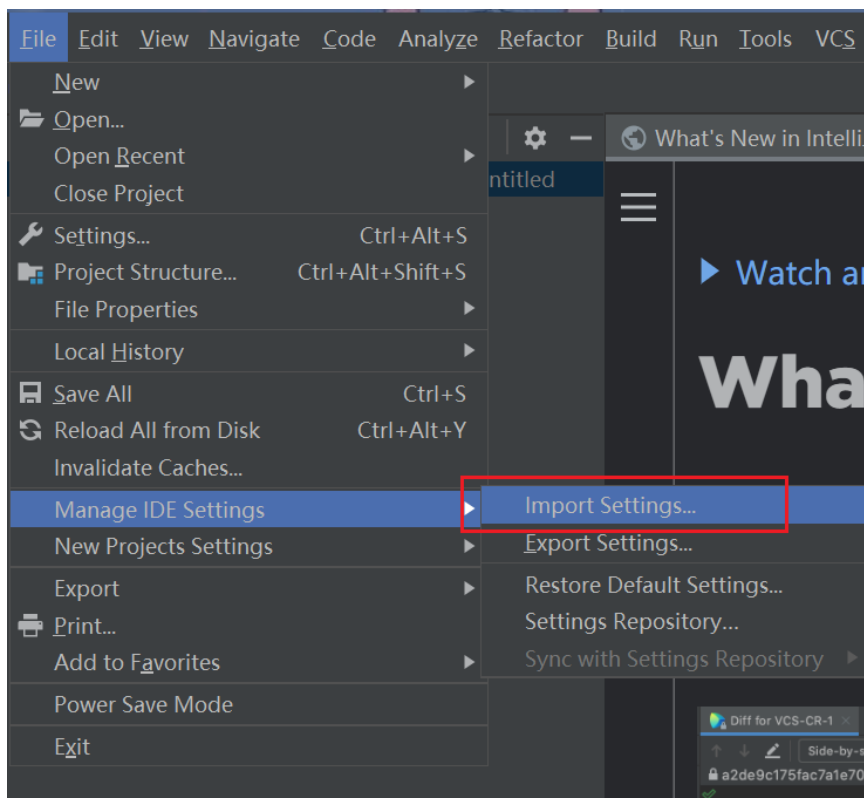
图 2.35 配置 IDEA
