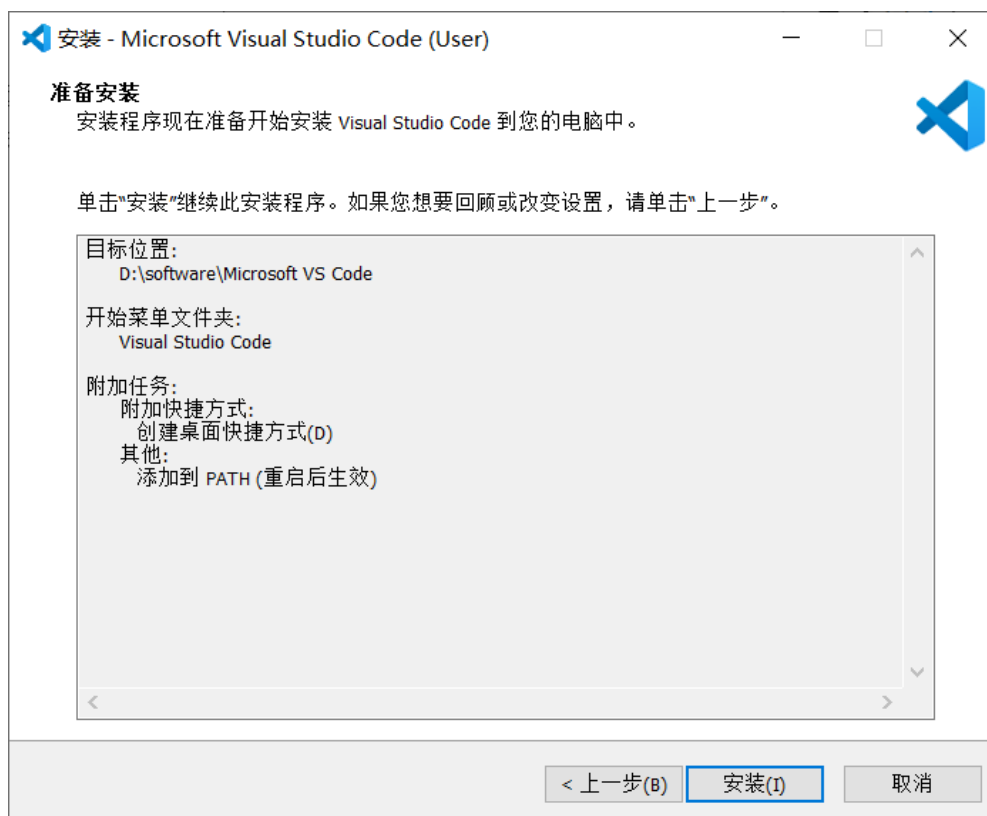
图 2.39 安装 VSCode
